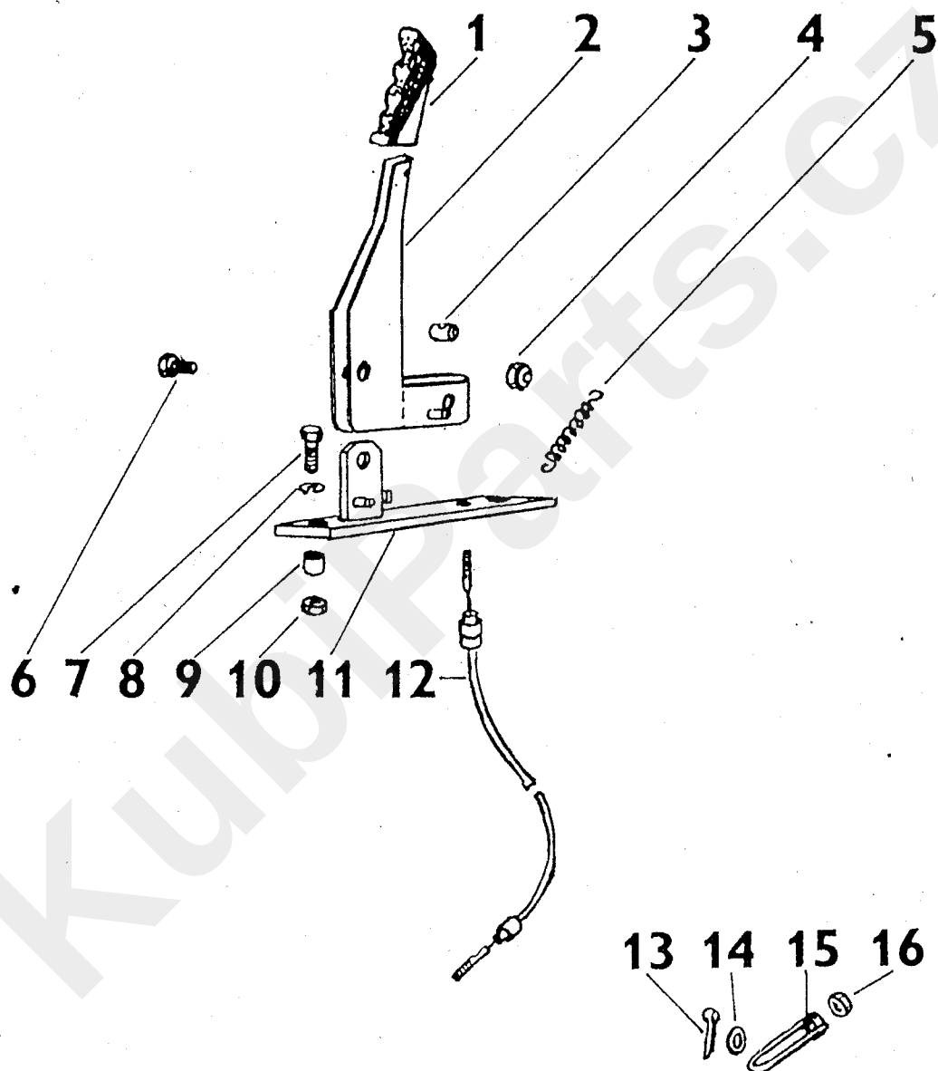
ZÁVĚS PRO JEDNONÁPRAVOVÝ PŘÍVĚS AUFHÄNGUNG FÜR EINACHSANHÄNGER - COUPLING FOR SEMI-TRAILER - ATTELAGE DE SEMI-REMORQUE
