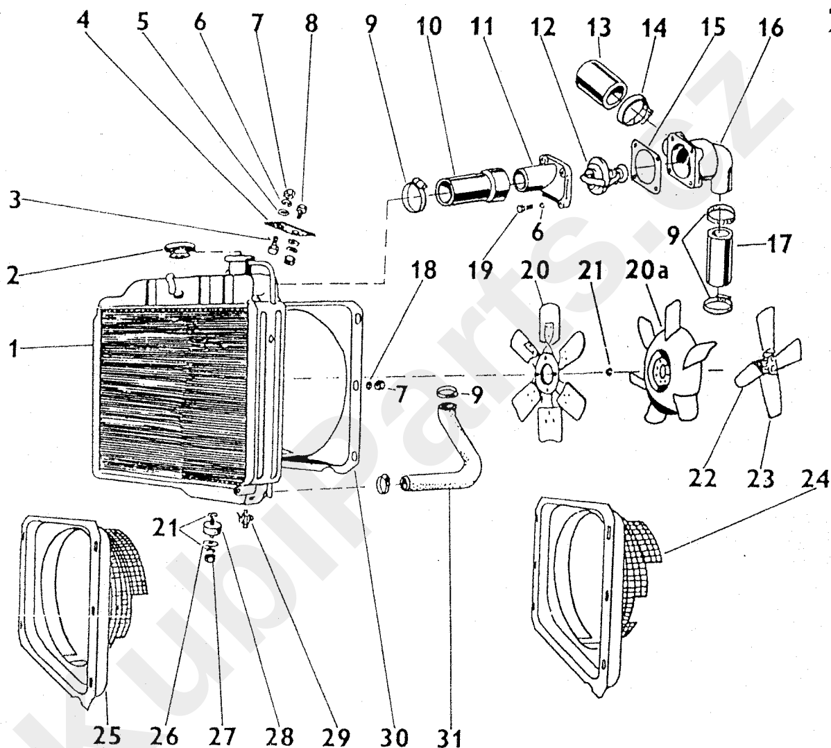
CHLADICÍ SYSTÉM KÜHLSYSTEM - COOLING SYSTEM - SYSTEME DE REFRIGERATION
