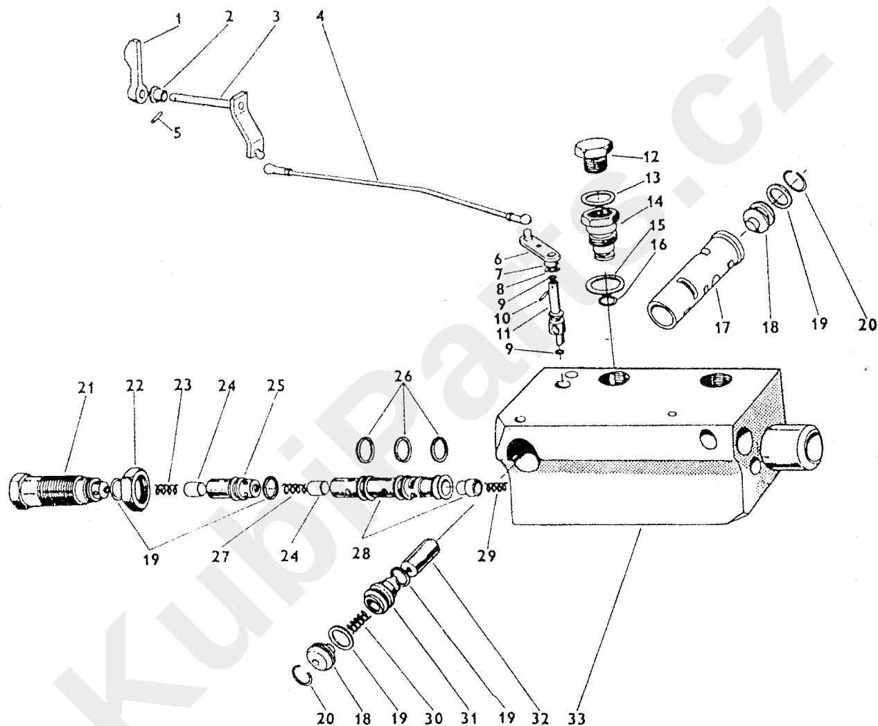
ROZVÁDĚČ VERTEILER - DISTRIBUTOR - DISTRIBUTEUR
