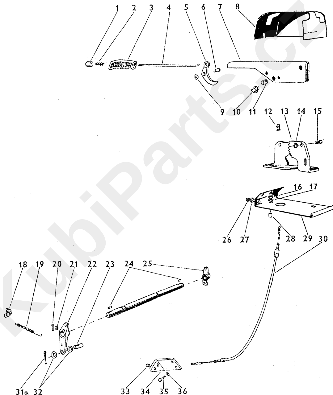
RUČNÍ BRZDA HANDBREMSE - HAND BRAKE - FREIN À MAIN
