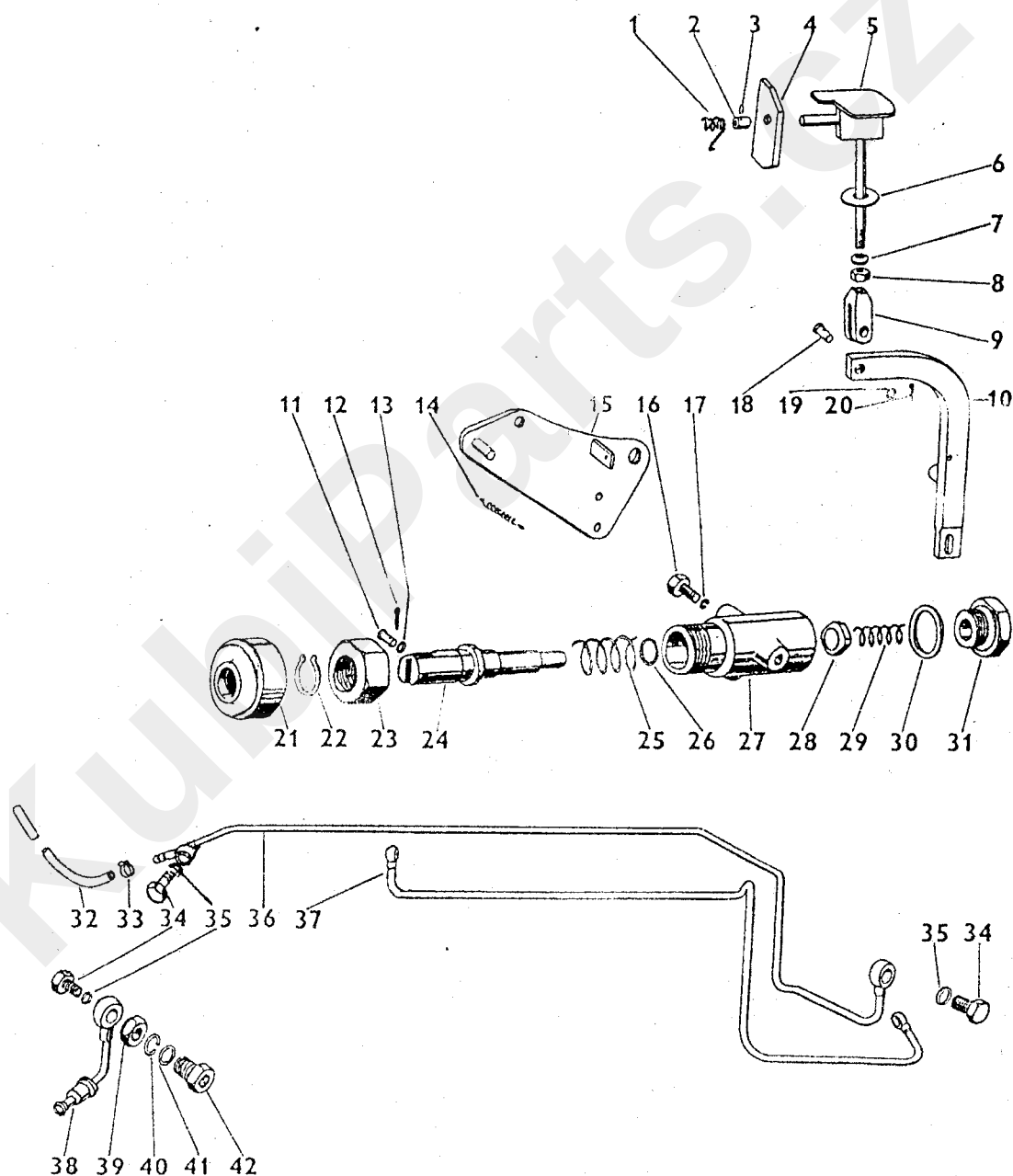
NÁSOBIČ TOČIVÉHO MOMENTU DREHMOMENTWANDLER - TORQUE CONVERTER - CONVERTISSEUR DU COUPLE
