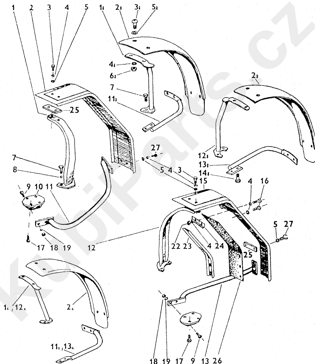
PŘEDNÍ BLATNÍKY - VORDERE KOTFLÜGEL - FRONT MUDGUARDS - AILES AVANT
