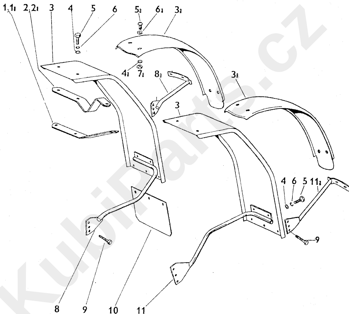
PŘEDNÍ BLATNÍKY VORDERE KOTFLÜGEL - FRONT MUDGUARDS - AILES AVANT
