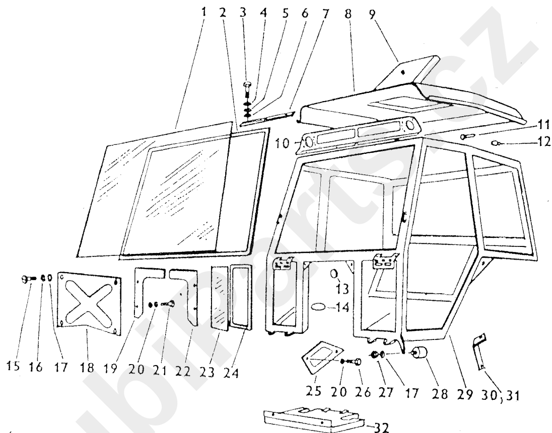
BEZPEČNOSTNÍ KABINA (BK 6011) SICHERHEITSKABINE - SAFETY CAB - CABINE DE SURETÉ
